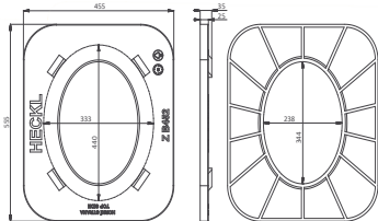
Deska hydrantová
